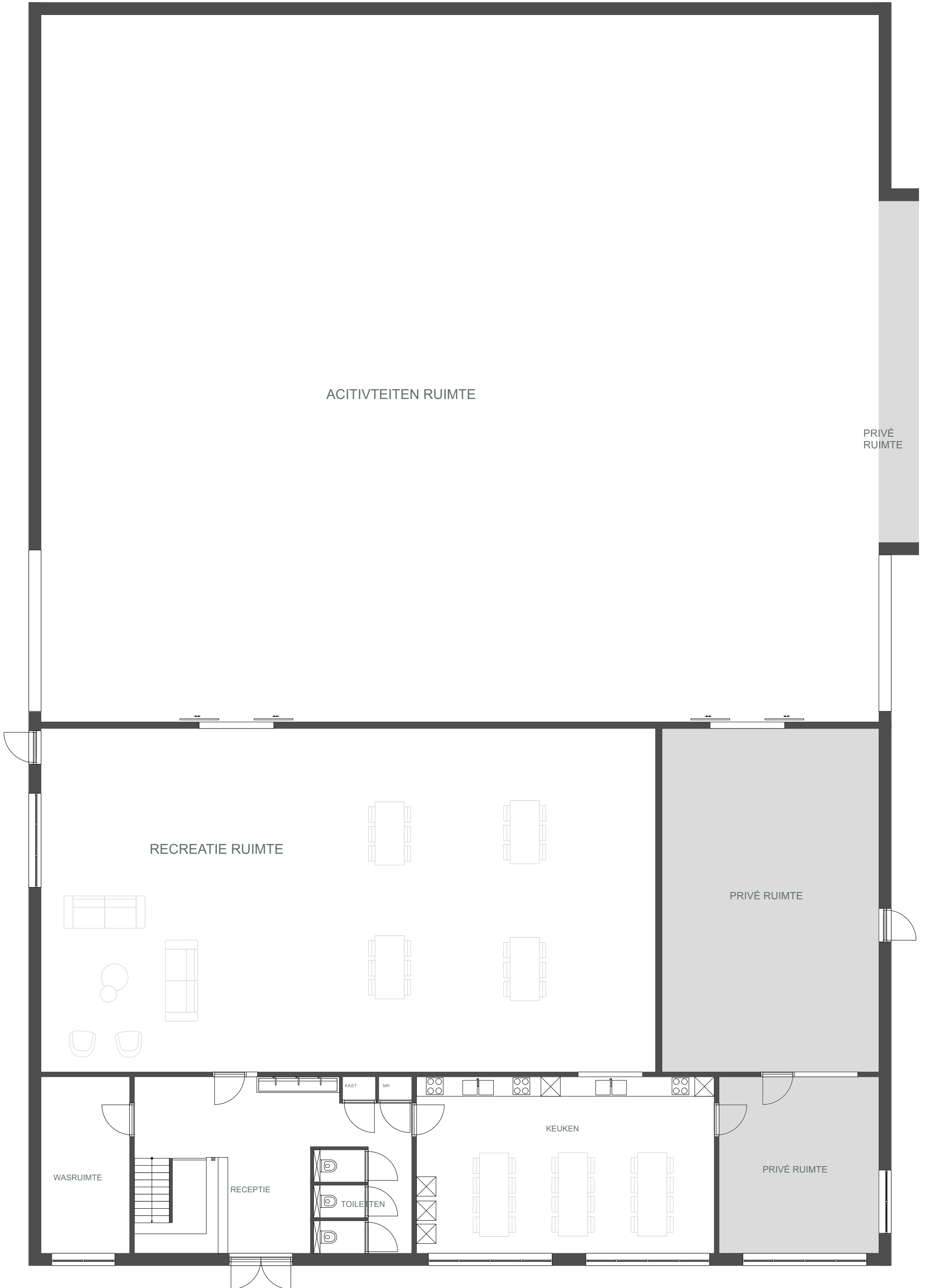
PLATTEGROND BEGANE GROND HOF VAN KESSEL
